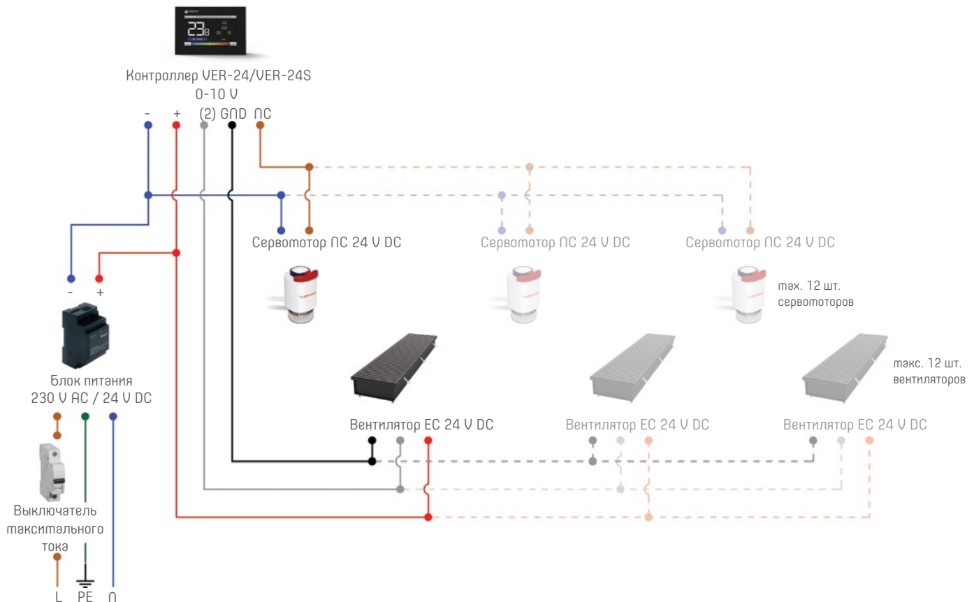
Пример схемы подключения одного или нескольких канальных нагревателей с вентилятором с использованием одного комнатного регулятора и приводов ON/OFF типа ПС
