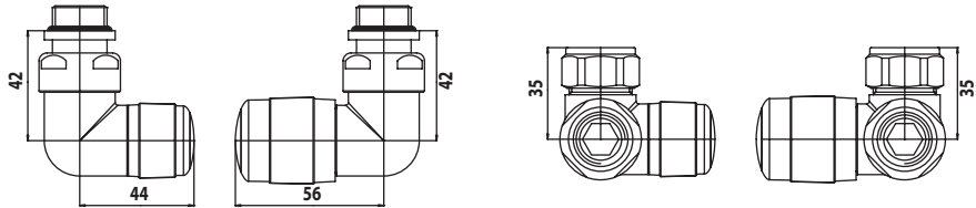
Комплект малогабаритных запорно-регулирующих вентилей - Рис. 7
