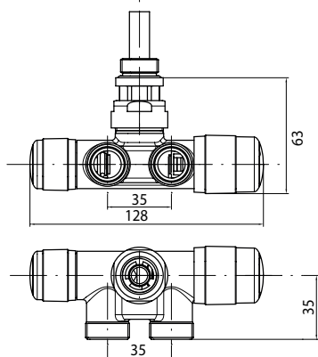
Комплект с термостатическим вентилем для углового однотрубного подключения (Рис. 14)
