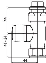
Комплект запорный и термостатический вентиль для прямого подключения Рис. 2
