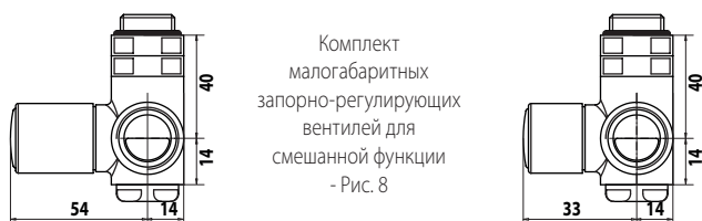
Комплект малогабаритных запорно-регулирующих вентилей для смешанной функции (Рис. 8)
