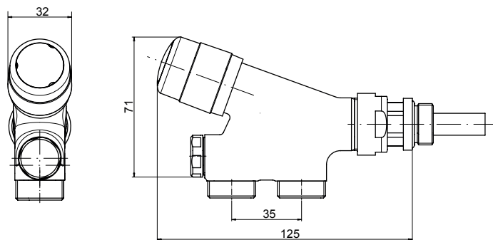
Комплект с термостатическим вентилем для углового однотрубного подключения (Рис. 14)
